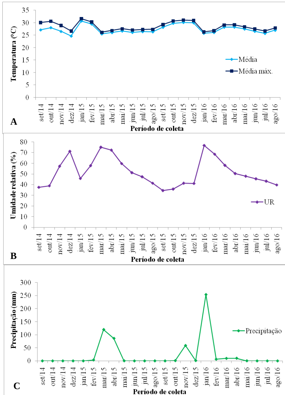
Figura 23: Dados climáticos do município de São Raimundo Nonato-PI ao longo do período de realização das coletas dos indivíduos: Temperatura média e média máxima (°C) (A); Umidade relativa do ar (UR) (B); Precipitação acumulada mensal (mm) (C).
